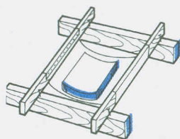
Travessas apoiadas no gabarito
